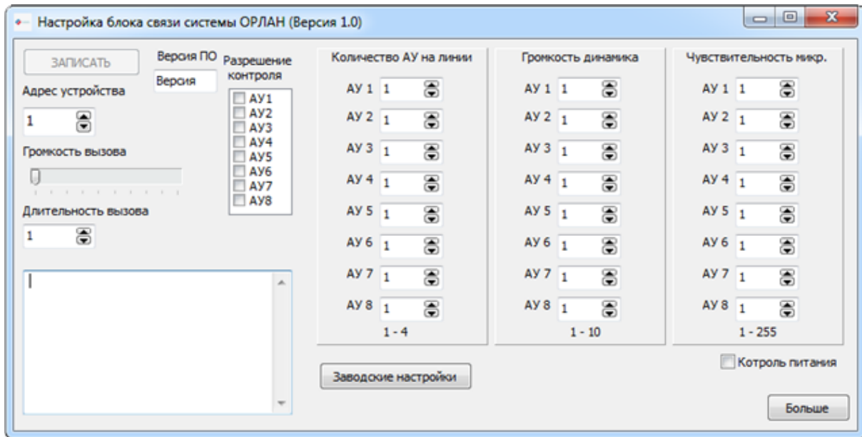
Рисунок 43. Окно программы настройки БС.
