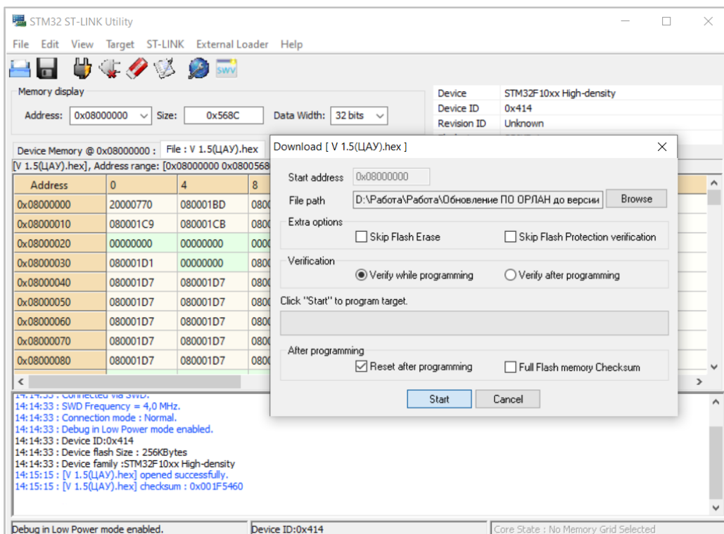
Рисунок 51. Окно выбора файла для обновления встроенного ПО в программе «STM32 ST-LINK Utility».
