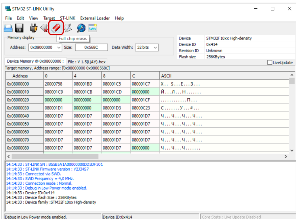
Рисунок 49. Кнопка «Full chip erase» программы «STM32 ST-LINK Utility».
