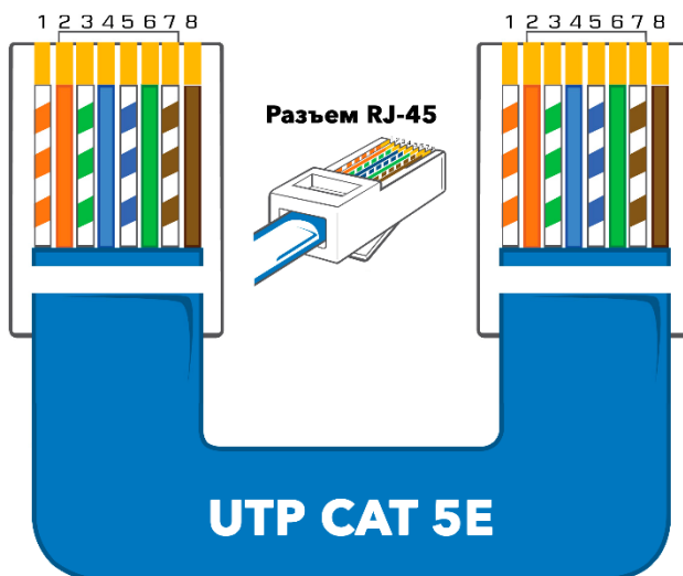
Рисунок 25. Схема подключения кабеля от БС МЕТА 17560/19560, БУ МЕТА 17661/19661 или соединительной коробки DR-2204 к МП МЕТА 18740-хх.
