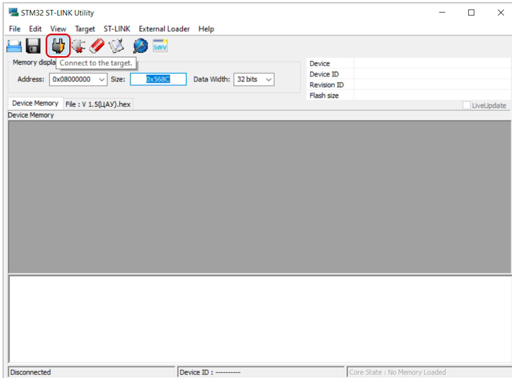
Рисунок 48. Основное окно программы «STM32 ST-LINK Utility» для обновления встроенного ПО.
