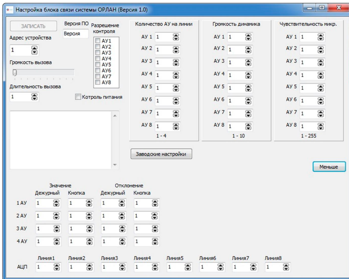
Рисунок 44. Окно программы настройки БС при нажатой кнопке «больше».
