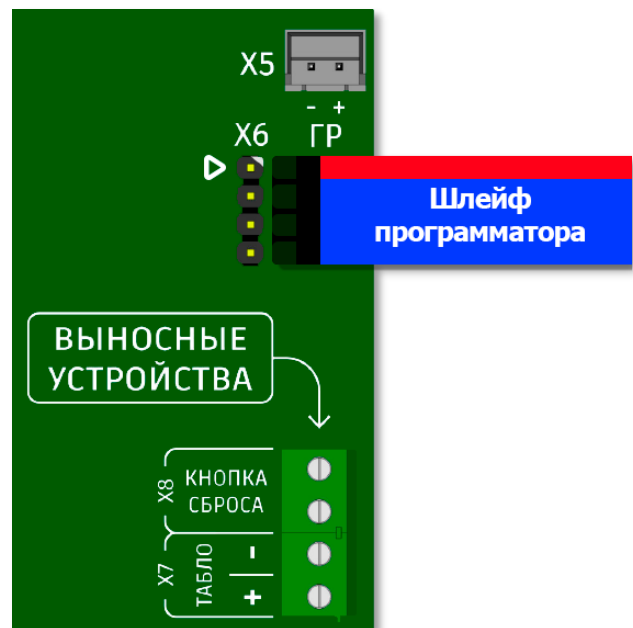
Рисунок 47. Подключение шлейфа программатора к ЦАУ МЕТА 18557 исп. В/В1/У/Н/МГН
